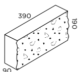
10.101 Full Length 14.3kg 108 per pallet 1544kg pallet weight
